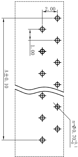
安装开孔
