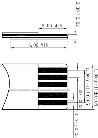
适用扁平电缆
